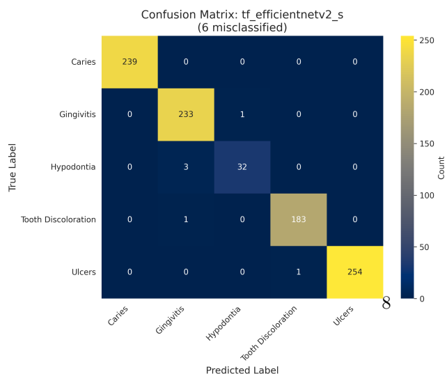
(q) EfficientNetV2-S (Baseline)
